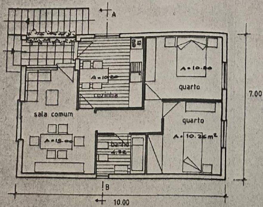
PLANTA DO ANDAR
