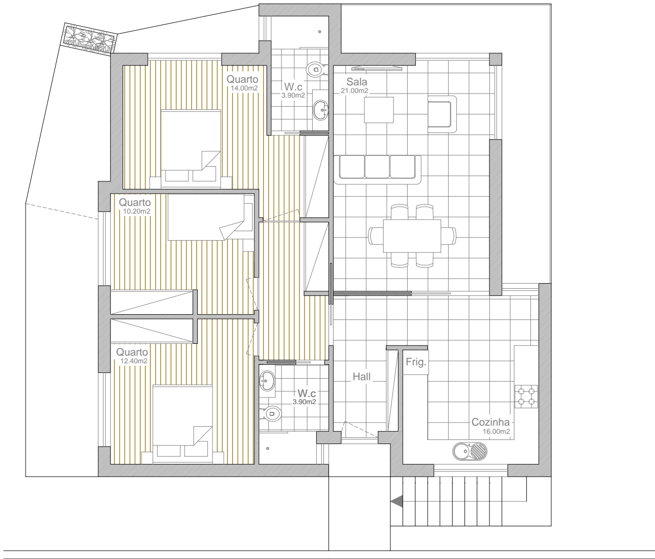
Planta do R/Chão
